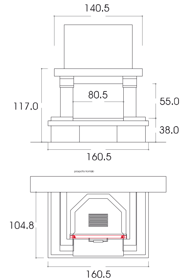
con interno: IDRO TERMO 80K25 TS cod. Arezzo 07
