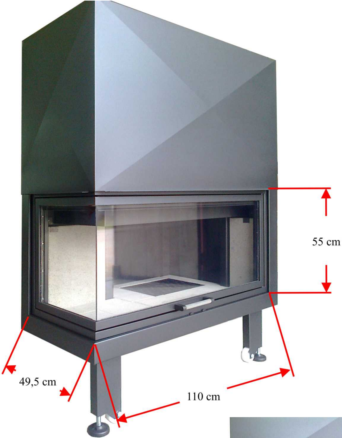
Termocamino ad acqua realizzato su misura Bocca da 110x49,5x55h
